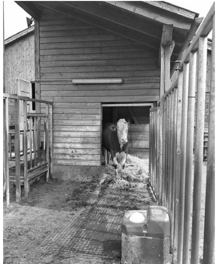
Über den Laufhof haben Kühe und Bullen die Möglichkeit, Kontakt aufzunehmen. Senkrechte Streben bilden eine stabile Einzäunung und ermöglichen dem Tierbetreuer gegebenenfalls die Flucht über die gesamte Länge der Deckbullenbucht.
